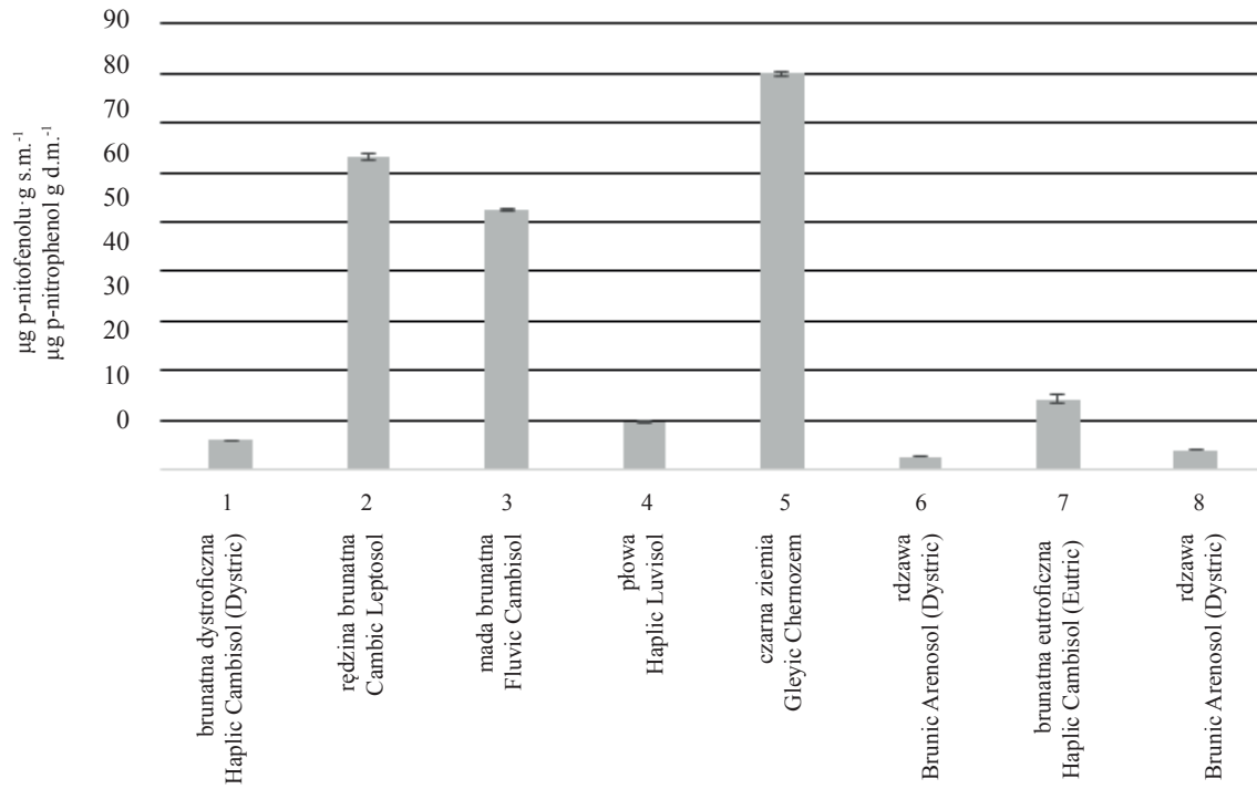
Rys. 8. Aktywność fosfatazy zasadowej w wierzchniej warstwie gleby (wartości średnie i odchylenia standardowe) Fig. 8. Alkaline phosphatase activity in topsoil as dependent. The means and standard deviations are presented.
