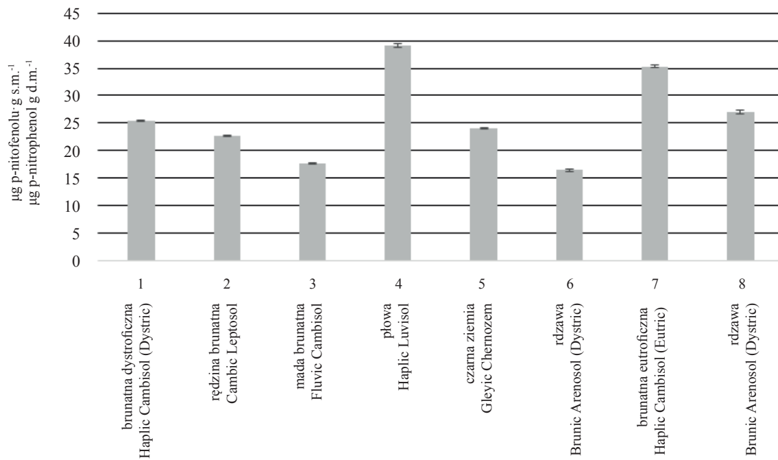
Rys. 9. Aktywność fosfatazy kwaśnej w wierzchniej warstwie gleby (wartości średnie i odchylenia standardowe) Fig. 9. Acidic phosphatase activity in topsoil. The means and standard deviations are presented.
