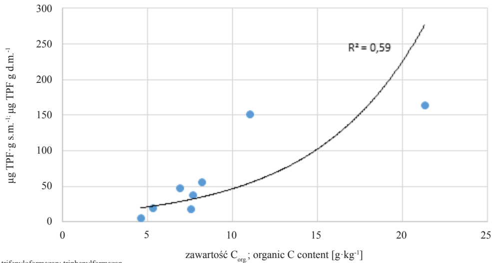
Rys. 12. Zależność między zawartością węgla organicznego w glebie a aktywnością dehydrogenaz Fig. 12. Relationship between organic carbon content in soil and dehydrogenase activity.
