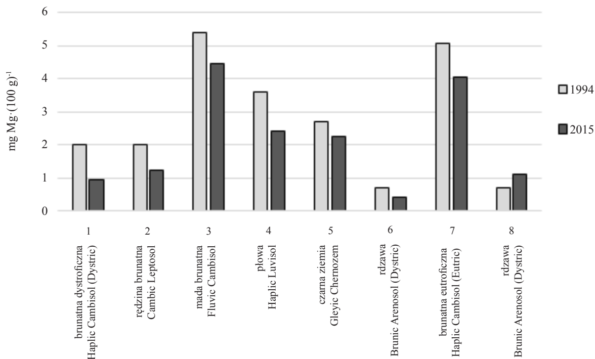
Rys. 5. Porównanie zawartości magnezu przyswajalnego w glebie w latach 1994 i 2015 Fig. 5. Comparison of soil available magnesium content between 1994 and 2015.
