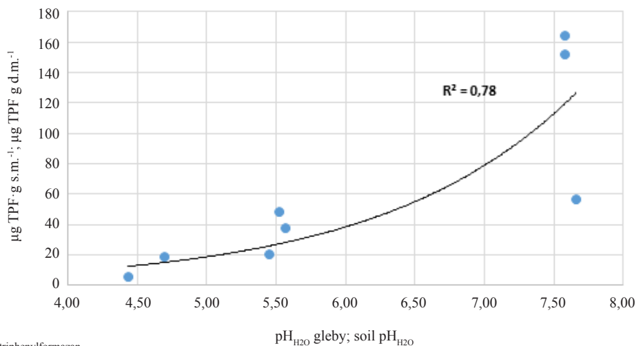
Rys. 10. Zależność między odczynem gleby a aktywnością dehydrogenaz
