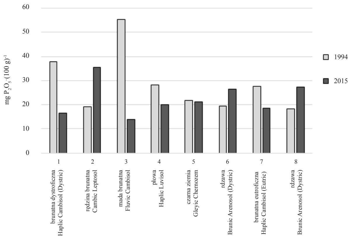
Rys. 3. Porównanie zawartości fosforu przyswajalnego w glebie w latach 1994 i 2015 Fig. 3. Comparison of soil available phosphorus content between 1994 and 2015.
