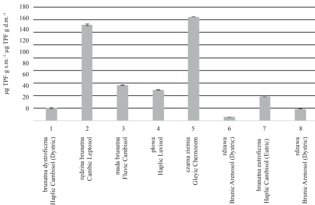
Rys. 7. Aktywność dehydrogenaz w wierzchniej warstwie gleby (wartości średnie i odchylenia standardowe) Fig. 7. Dehydrogenases activity in topsoil. The means and standard deviations are presented.
