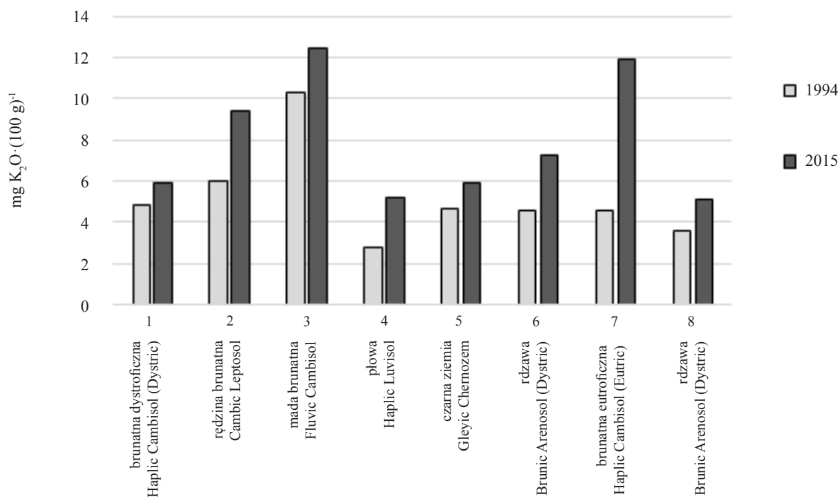
Rys. 4. Porównanie zawartości potasu przyswajalnego w glebie w latach 1994 i 2015 Fig. 4. Comparison of soil available potassium content between 1994 and 2015.
