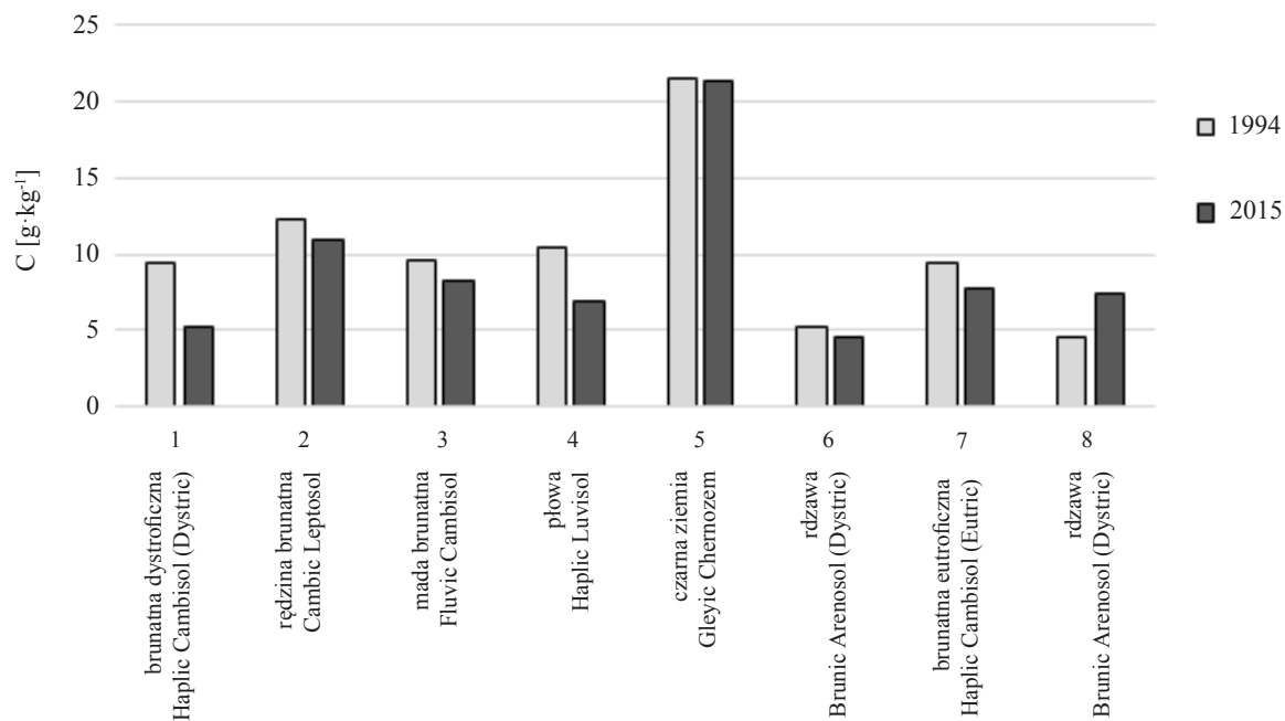
Rys. 2. Porównanie zawartości węgla w glebie w latach 1994 i 2015 Fig. 2. Comparison of soil C content between 1994 and 2015.
